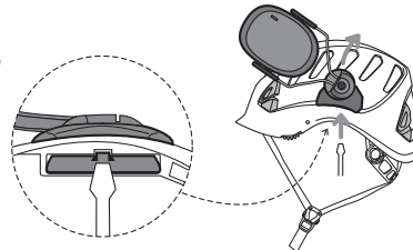
Removing Déclippage
