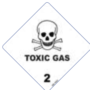
QSI 3844 D 1 D 3 D 4 D 6 D 8 D 9
