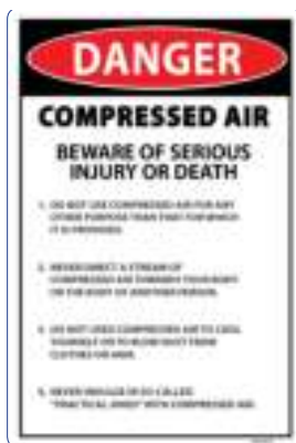
QSI 3639 H 1 H 3 H 4 H 5 H 6 H 7 H 8
