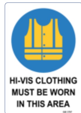
QSI 3787 F 1 F 3 F 4 F 5 F 6 F 7 F 8 H 3 H 4 H 5 H 6 H 7 H 8
